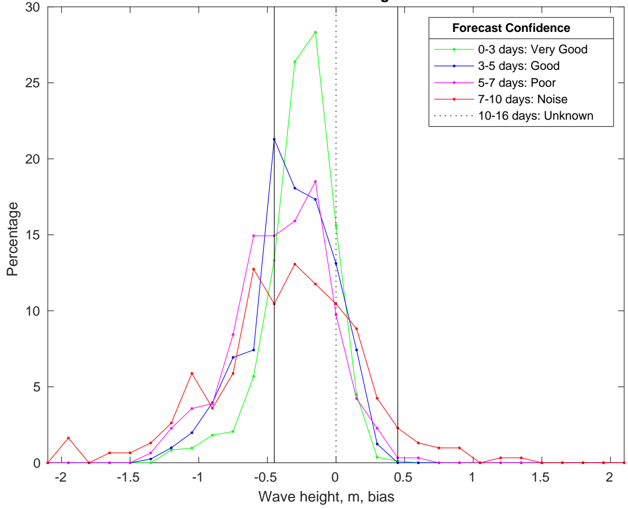
NDBC 42019 vs CMEMSWaves Bias Histogram: 09-Jan-2025
