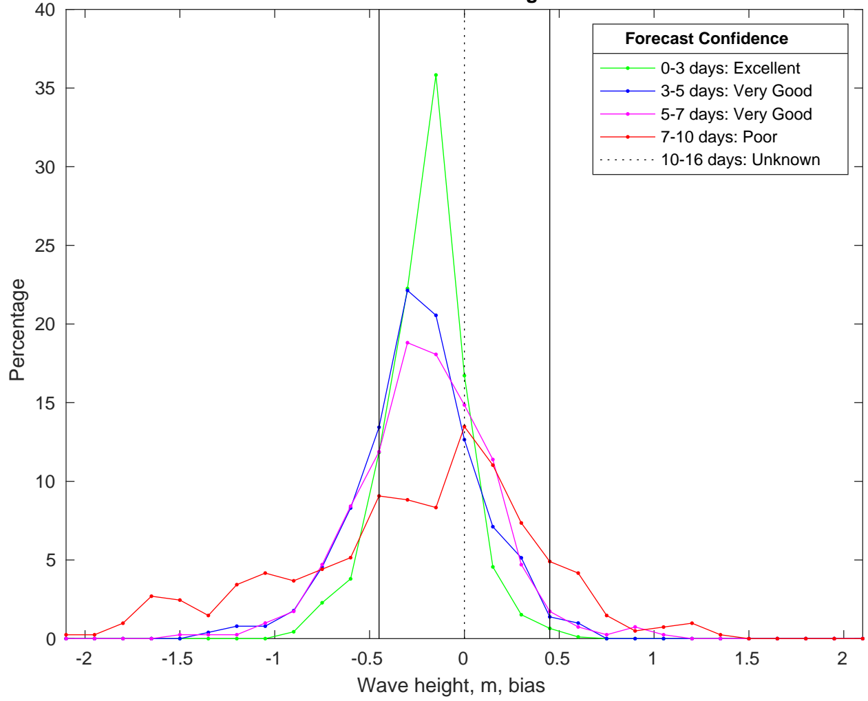
NDBC 42036 vs CMEMSWaves Bias Histogram: 12-Jan-2025
