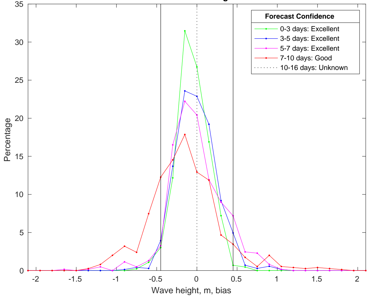
NDBC 46054 vs CMEMSWaves Bias Histogram: 20-Jan-2025
