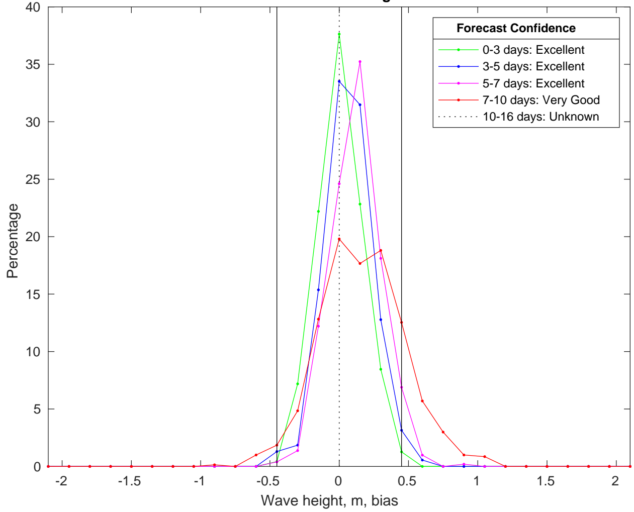
NDBC 41040 vs CMEMSWaves Bias Histogram: 02-Feb-2025
