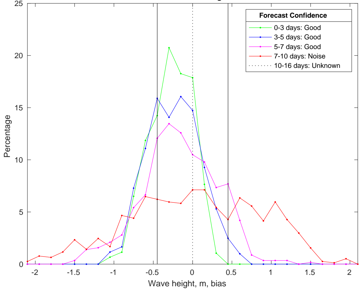
NDBC 42019 vs CMEMSWaves Bias Histogram: 02-Feb-2025
