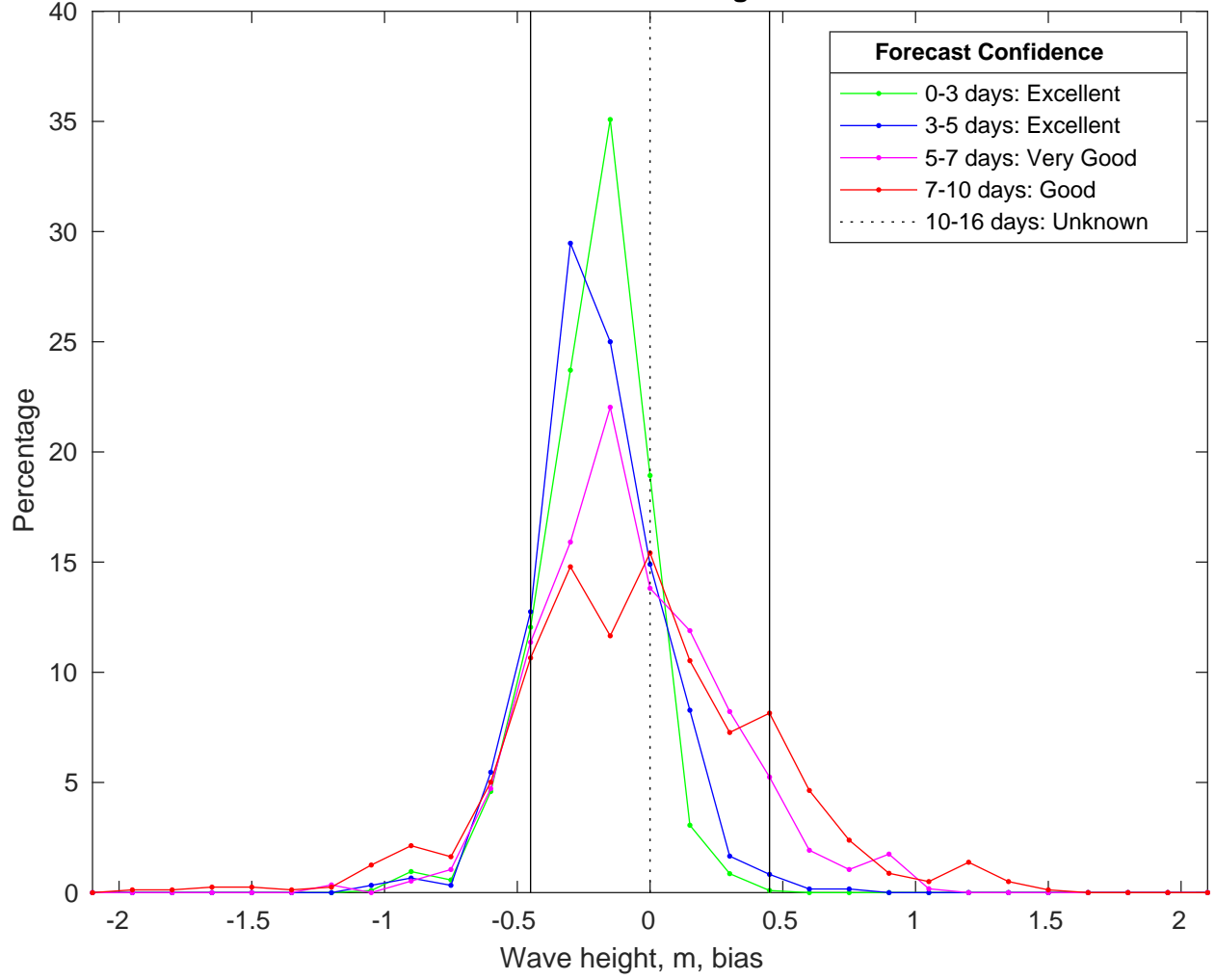
NDBC 42036 vs CMEMSWaves Bias Histogram: 02-Feb-2025
