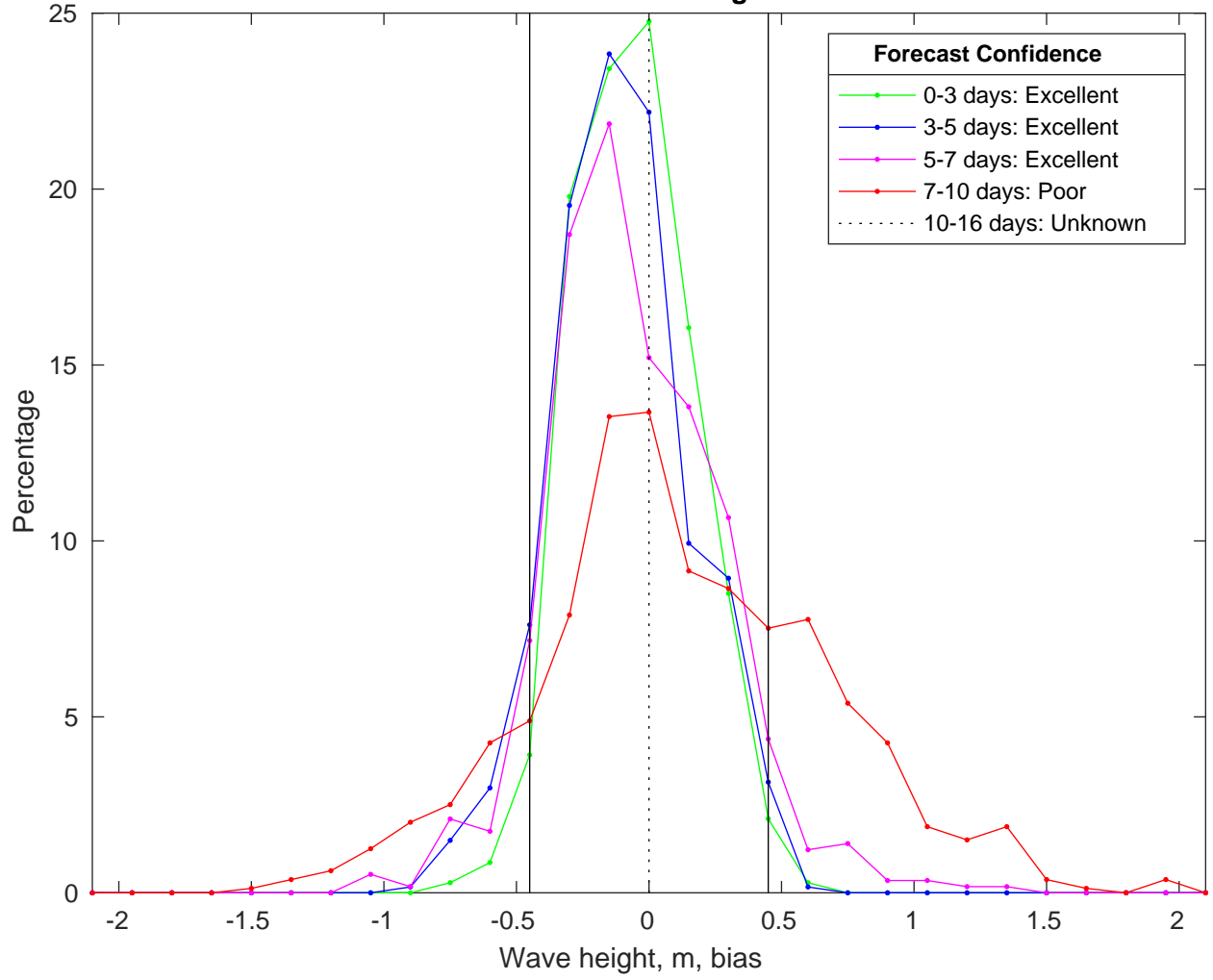
NDBC 42084 vs CMEMSWaves Bias Histogram: 02-Feb-2025
