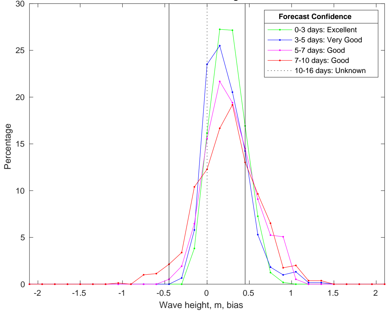
NDBC 44020 vs CMEMSWaves Bias Histogram: 02-Feb-2025
