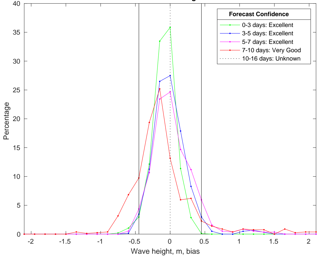
NDBC 46054 vs CMEMSWaves Bias Histogram: 02-Feb-2025
