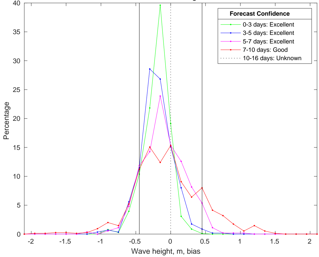
NDBC 42036 vs CMEMSWaves Bias Histogram: 03-Feb-2025
