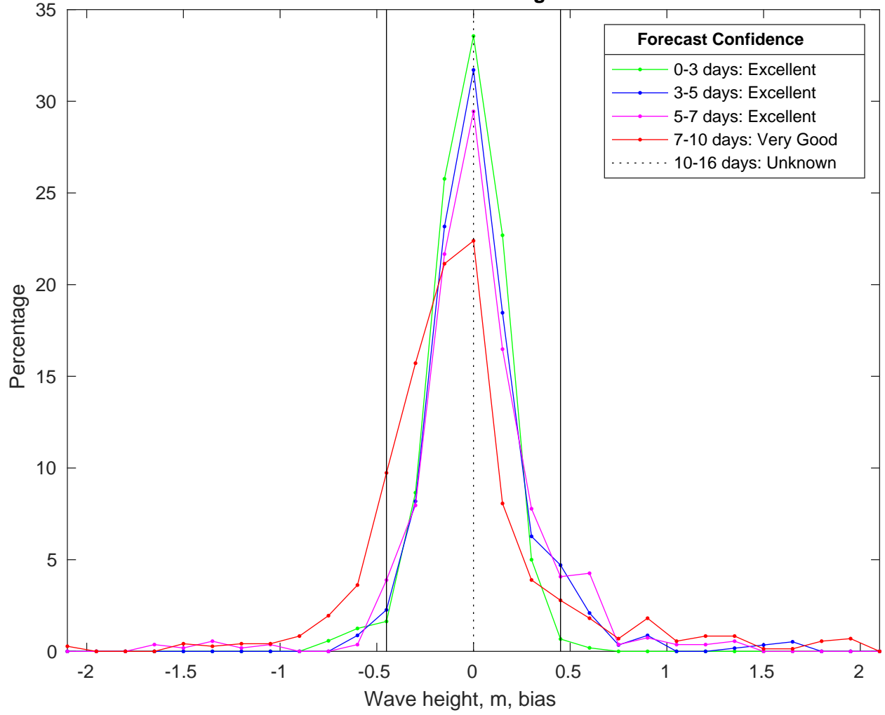
NDBC 46028 vs CMEMSWaves Bias Histogram: 03-Feb-2025
