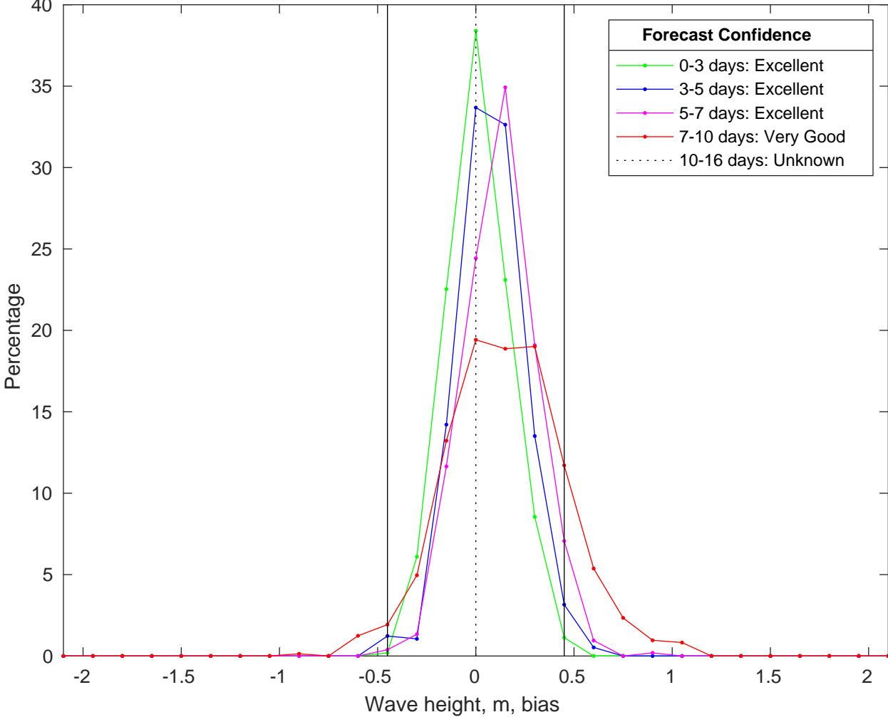
NDBC 41040 vs CMEMSWaves Bias Histogram: 04-Feb-2025
