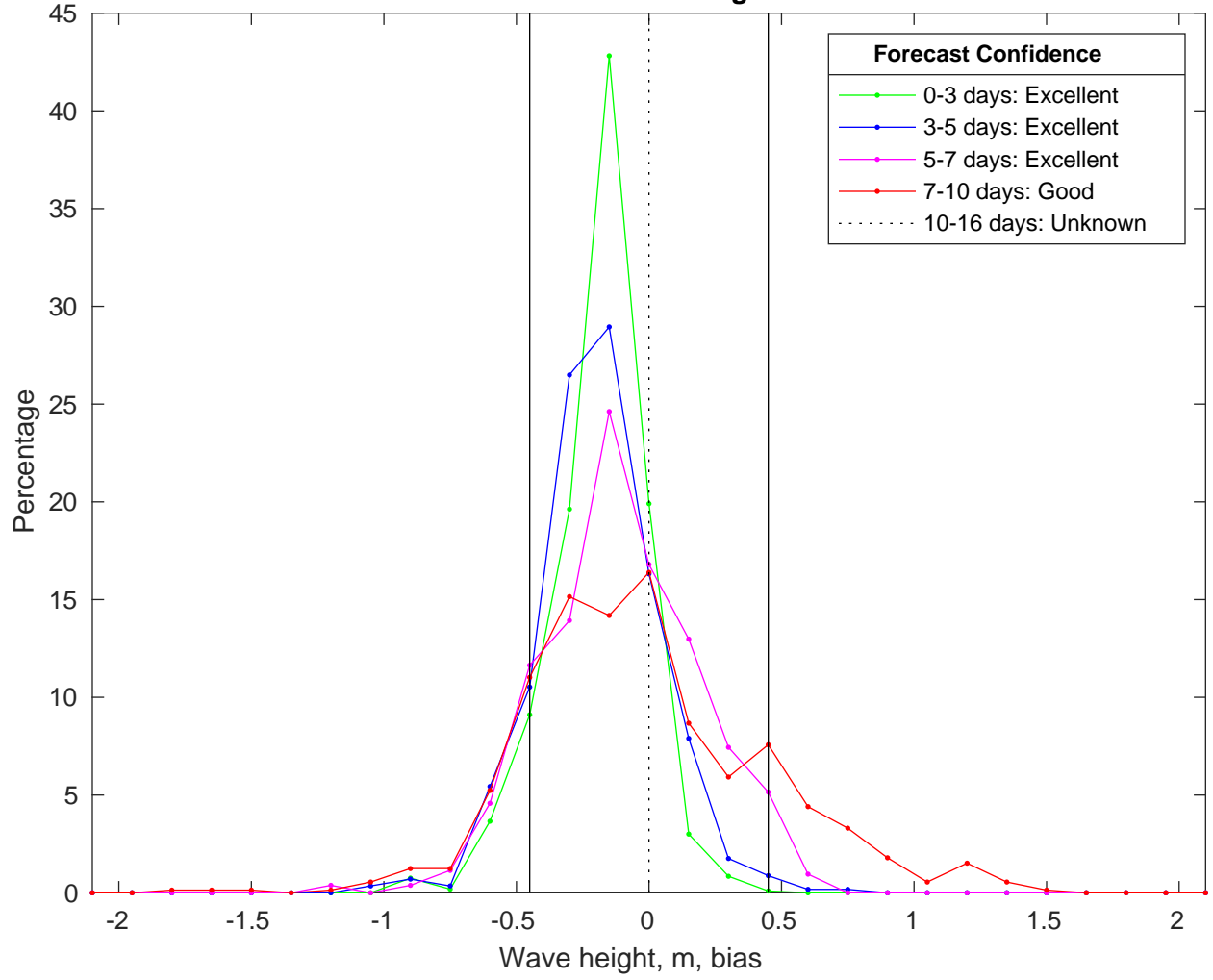
NDBC 42036 vs CMEMSWaves Bias Histogram: 04-Feb-2025
