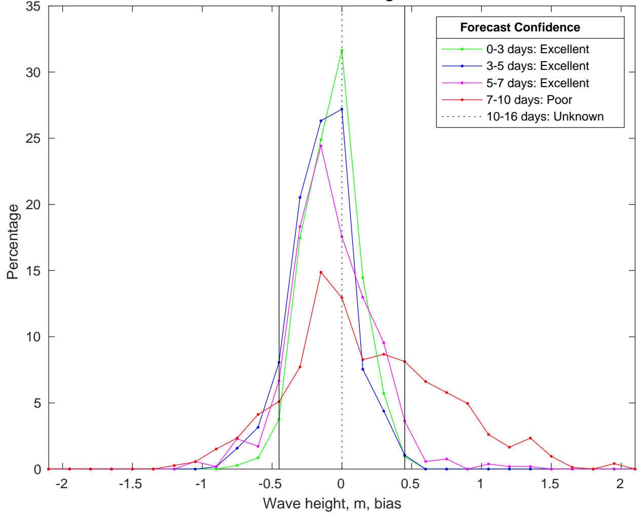
NDBC 42084 vs CMEMSWaves Bias Histogram: 04-Feb-2025
