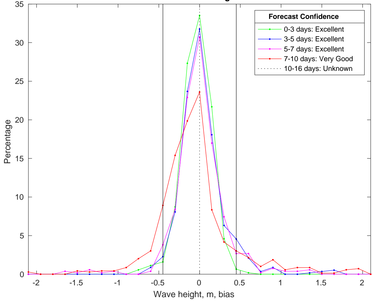
NDBC 46028 vs CMEMSWaves Bias Histogram: 04-Feb-2025
