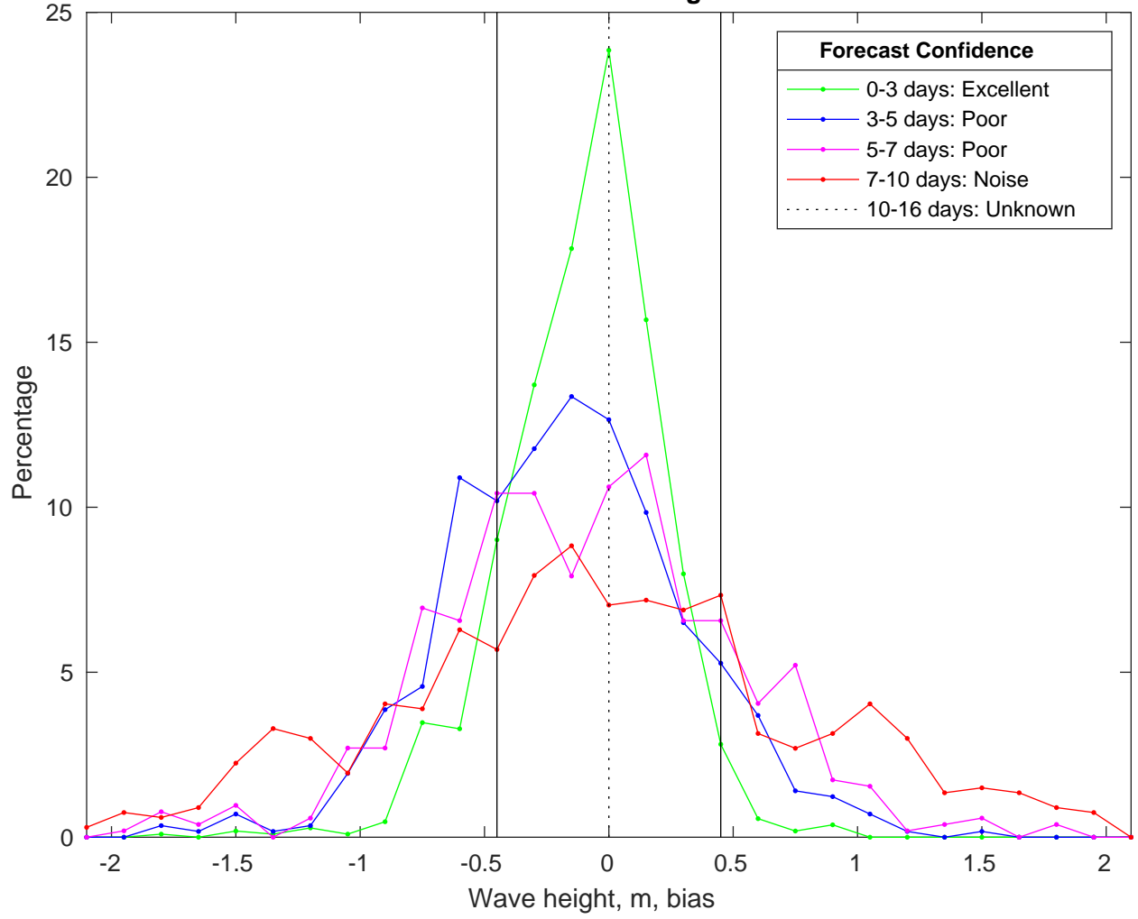
NDBC 46246 vs CMEMSWaves Bias Histogram: 04-Feb-2025
