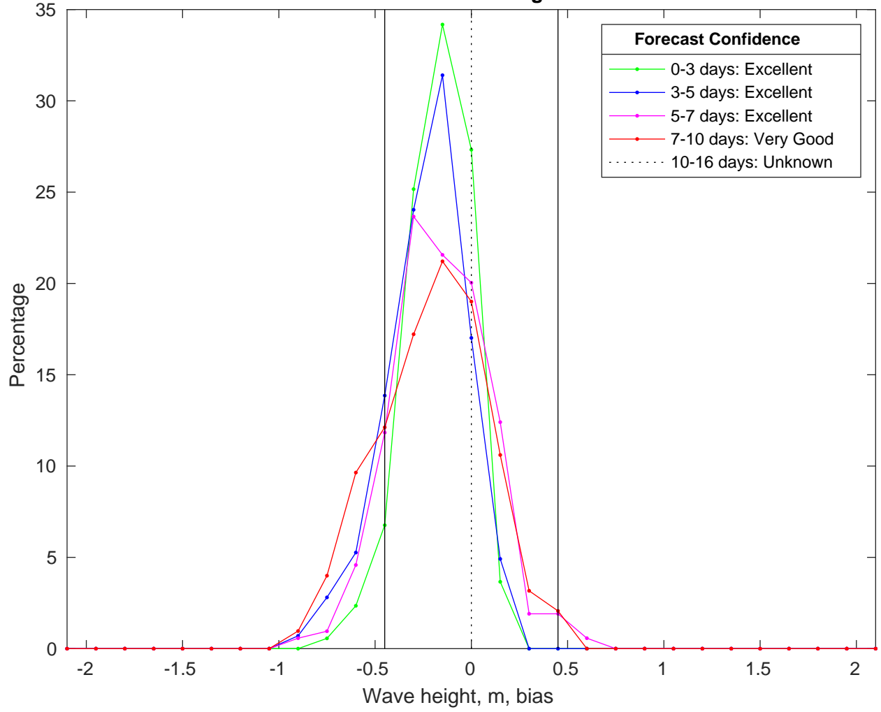
NDBC 52211 vs CMEMSWaves Bias Histogram: 04-Feb-2025
