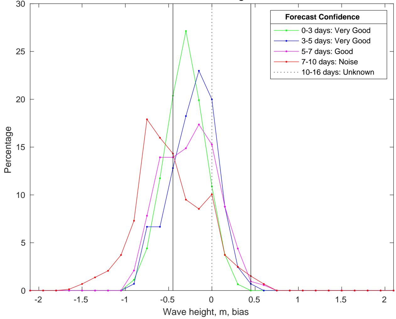
NDBC 52213 vs CMEMSWaves Bias Histogram: 04-Feb-2025
