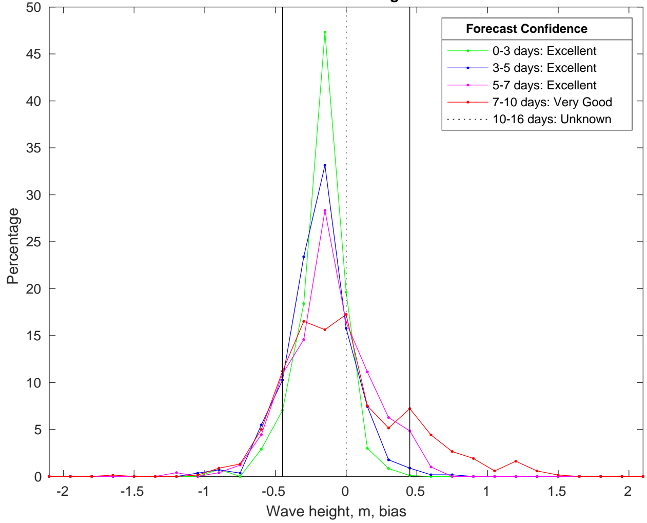
NDBC 42036 vs CMEMSWaves Bias Histogram: 05-Feb-2025
