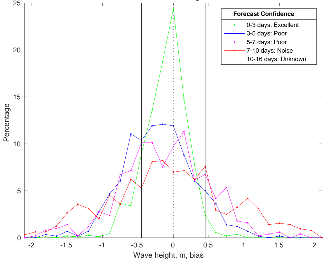
NDBC 46246 vs CMEMSWaves Bias Histogram: 05-Feb-2025
