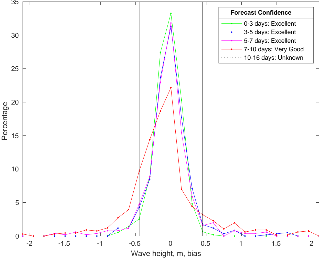
NDBC 46028 vs CMEMSWaves Bias Histogram: 05-Feb-2025
