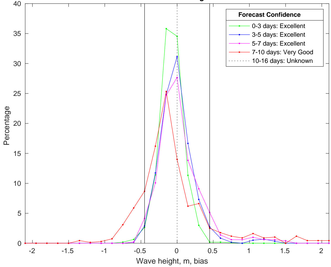
NDBC 46054 vs CMEMSWaves Bias Histogram: 05-Feb-2025
