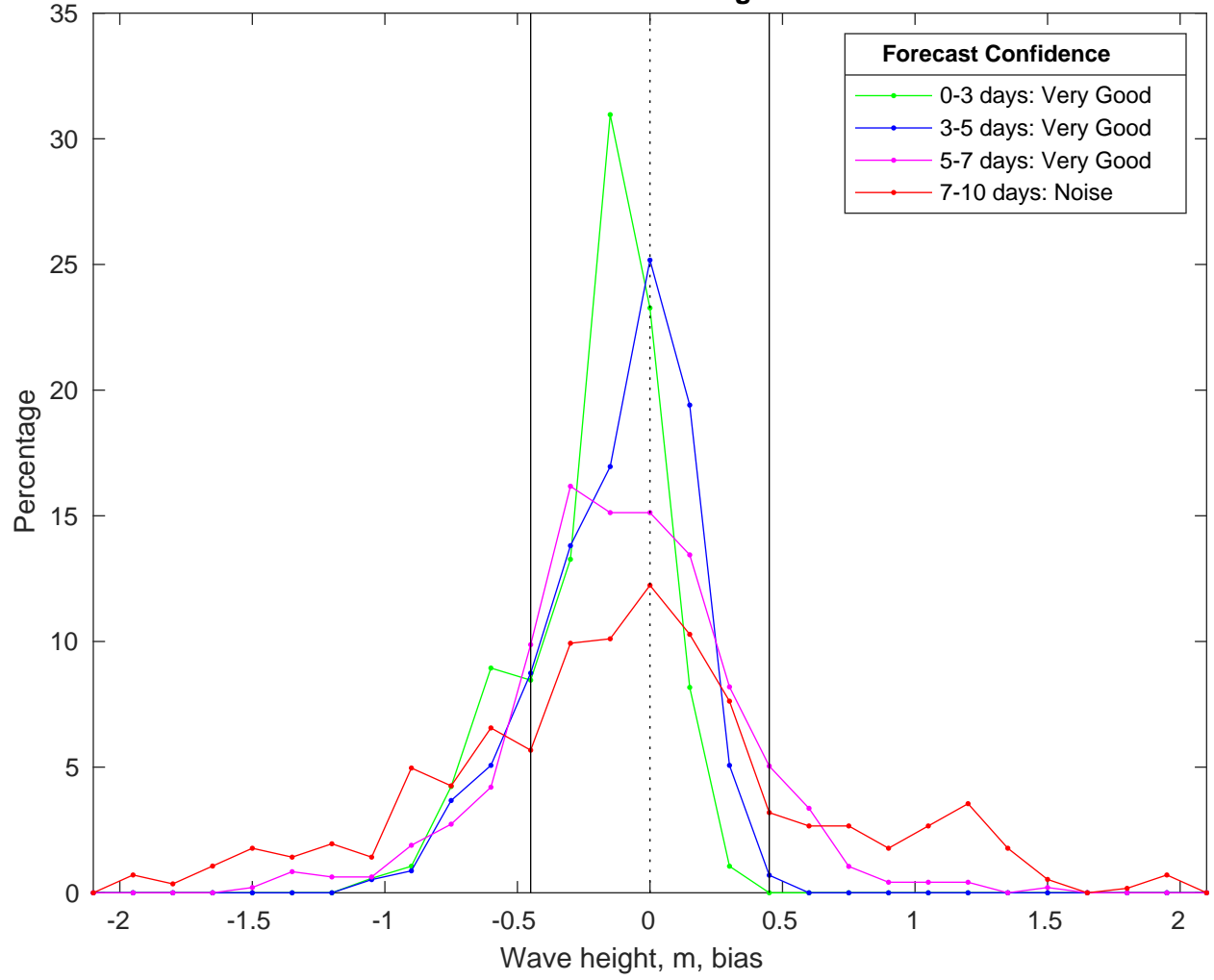
NDBC 42019 vs CMEMS Waves Bias Histogram: 07-Feb-2025
