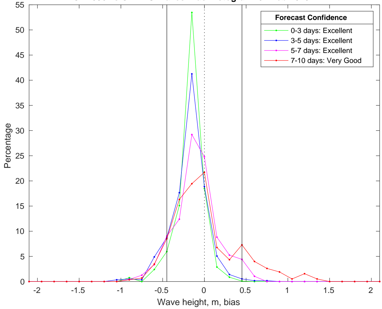
NDBC 42036 vs CMEMS Waves Bias Histogram: 07-Feb-2025
