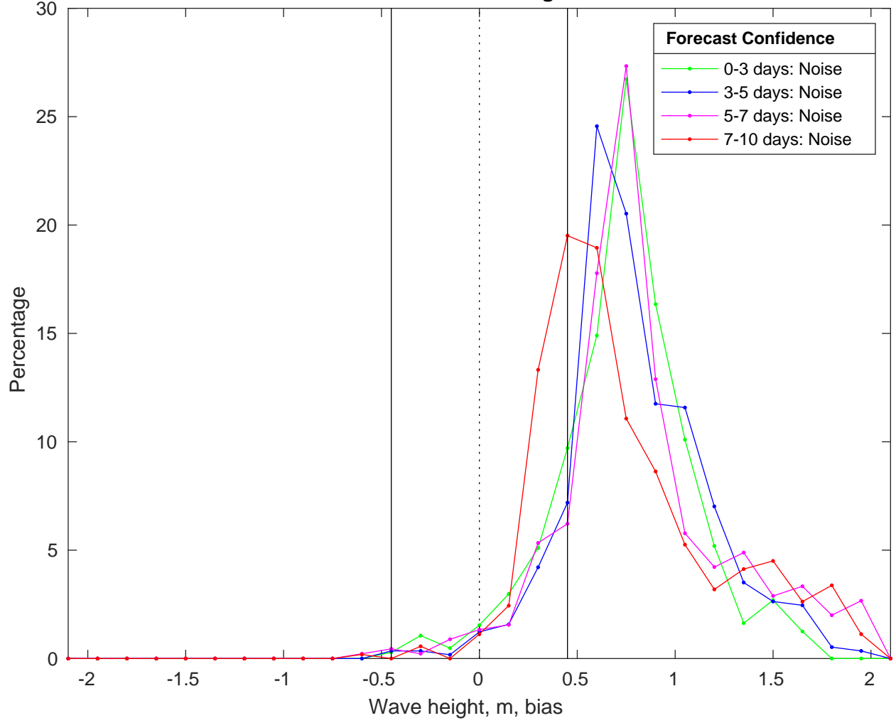
NDBC 46053 vs CMEMS Waves Bias Histogram: 07-Feb-2025
