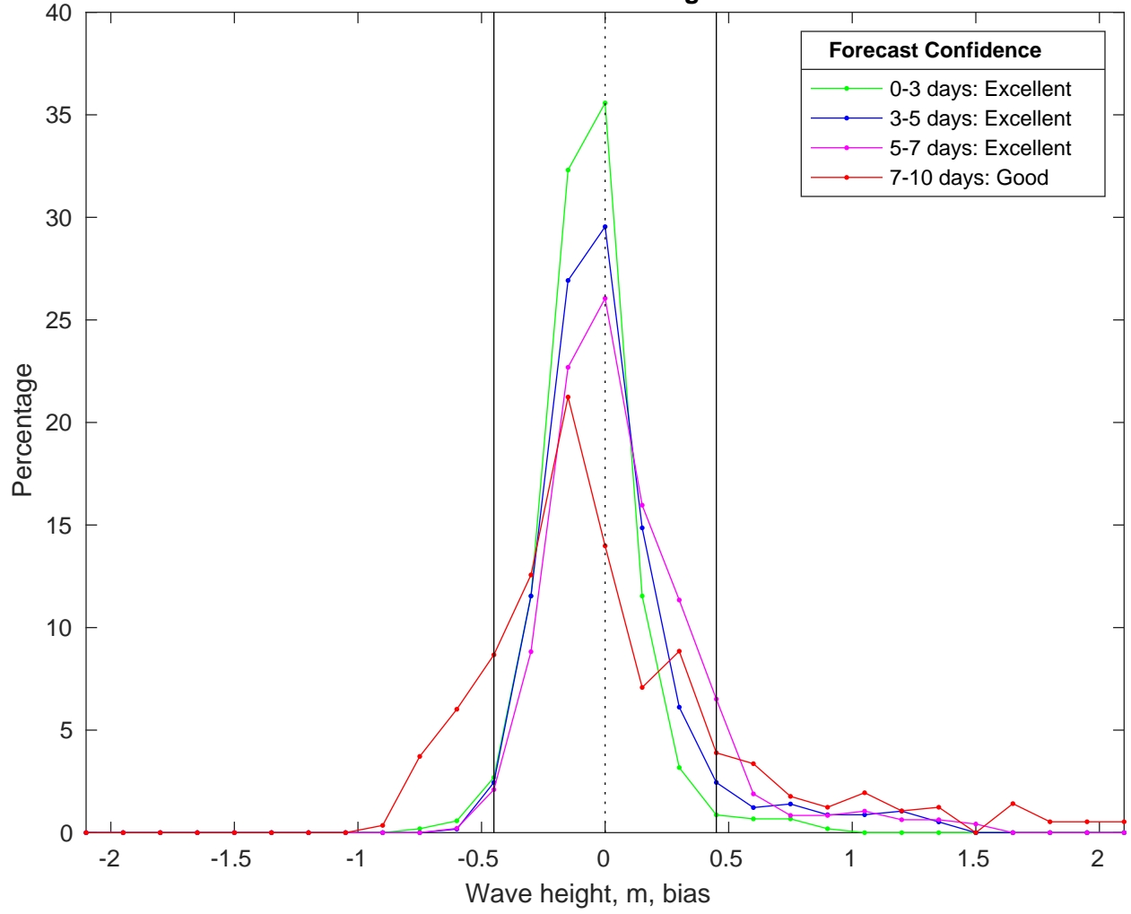
NDBC 46054 vs CMEMS Waves Bias Histogram: 07-Feb-2025
