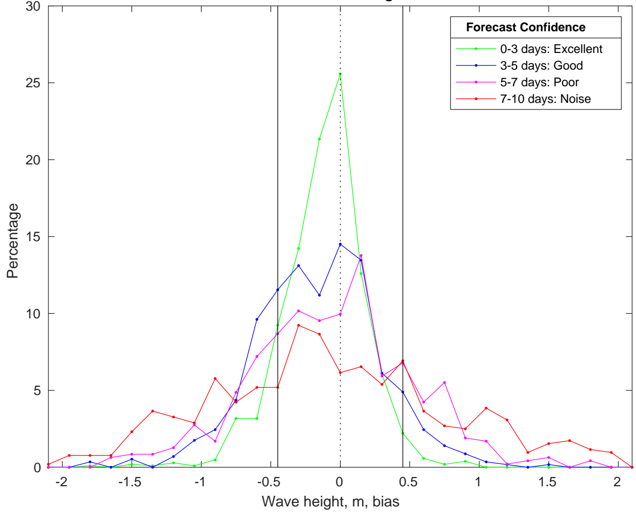
NDBC 46246 vs CMEMS Waves Bias Histogram: 07-Feb-2025
