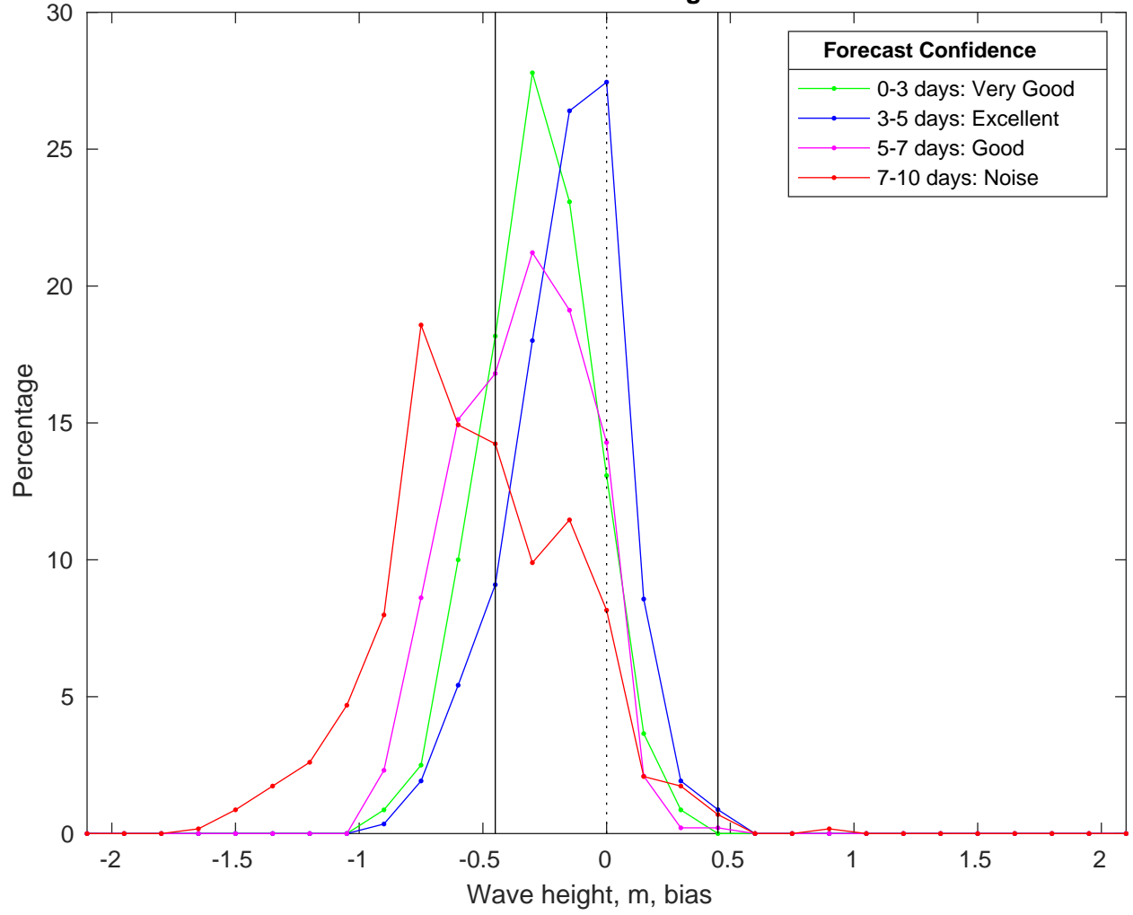
NDBC 52213 vs CMEMS Waves Bias Histogram: 07-Feb-2025
