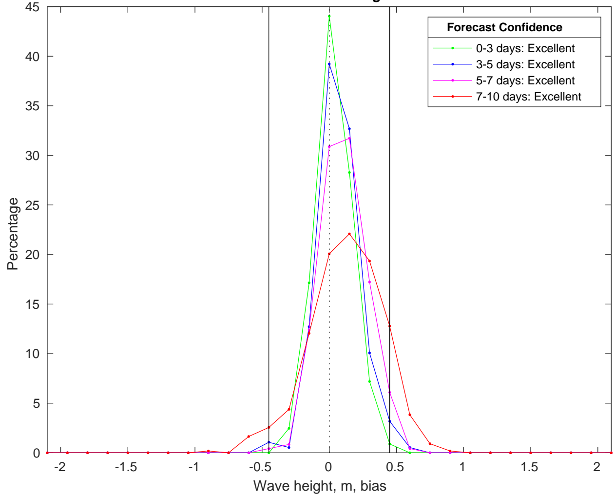
NDBC 41040 vs CMEMS Waves Bias Histogram: 08-Feb-2025
