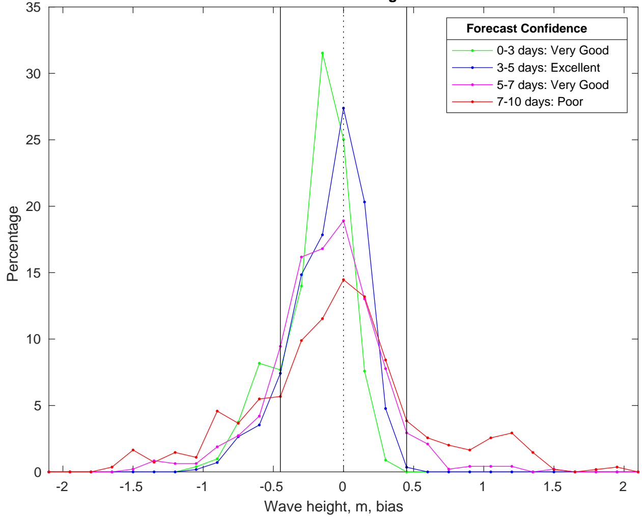
NDBC 42019 vs CMEMS Waves Bias Histogram: 08-Feb-2025
