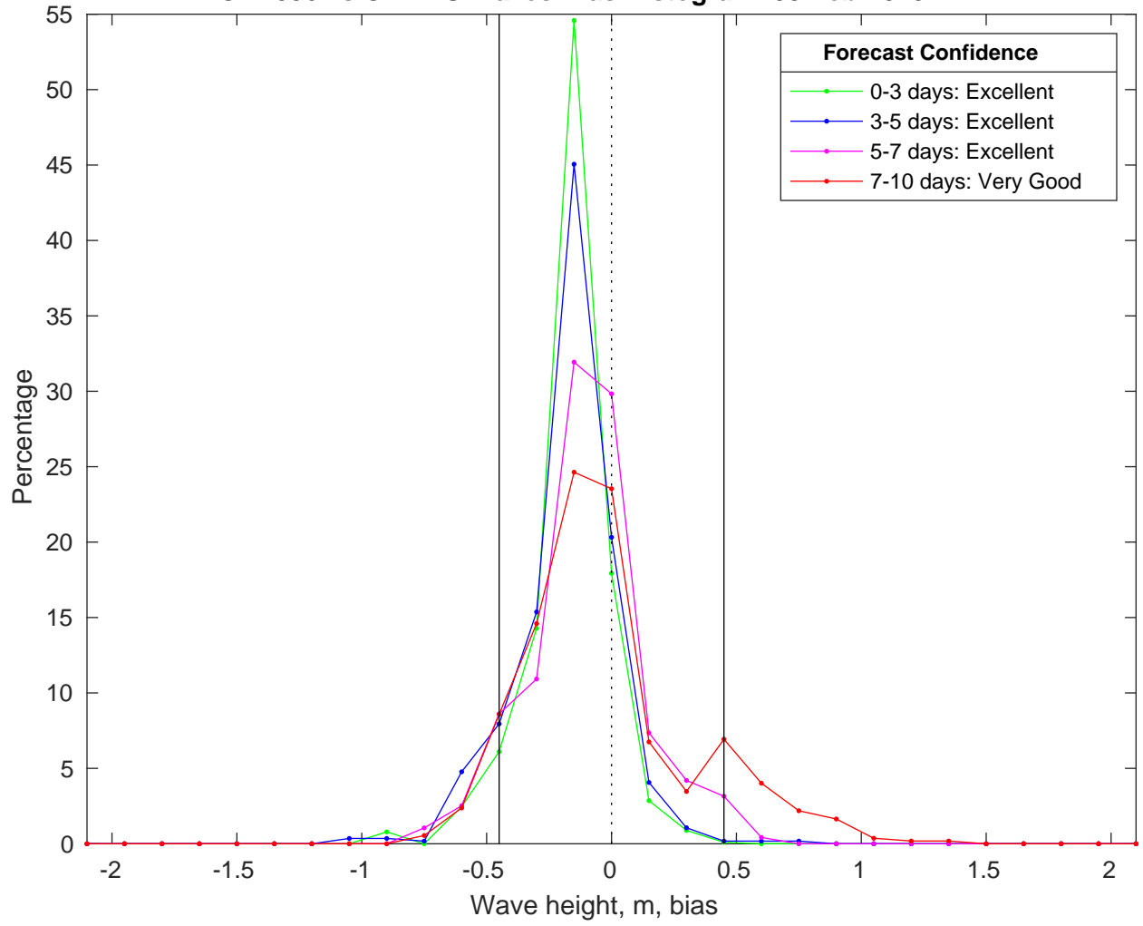
NDBC 42036 vs CMEMS Waves Bias Histogram: 08-Feb-2025
