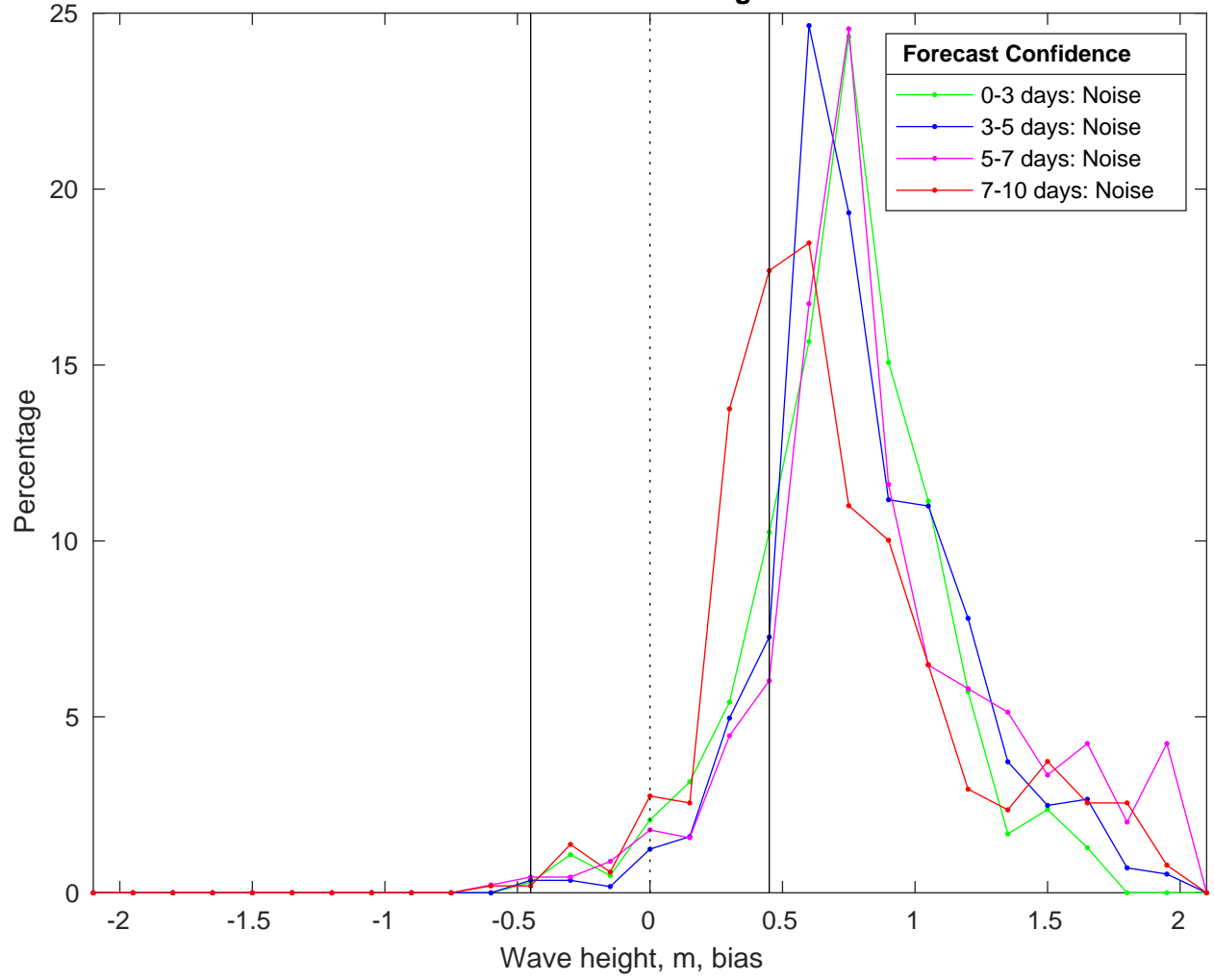
NDBC 46053 vs CMEMS Waves Bias Histogram: 08-Feb-2025
