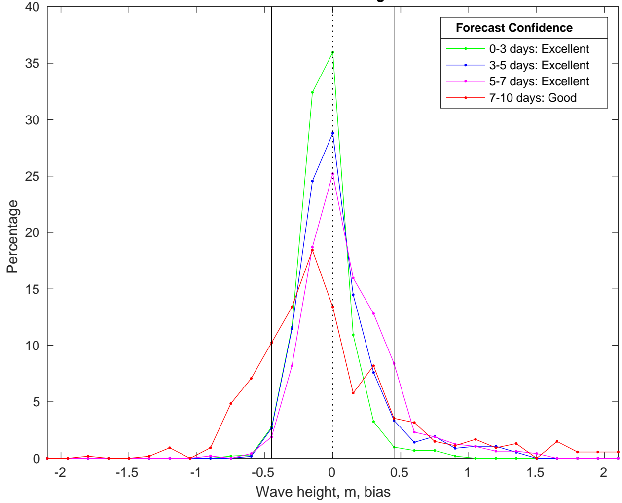
NDBC 46054 vs CMEMS Waves Bias Histogram: 08-Feb-2025
