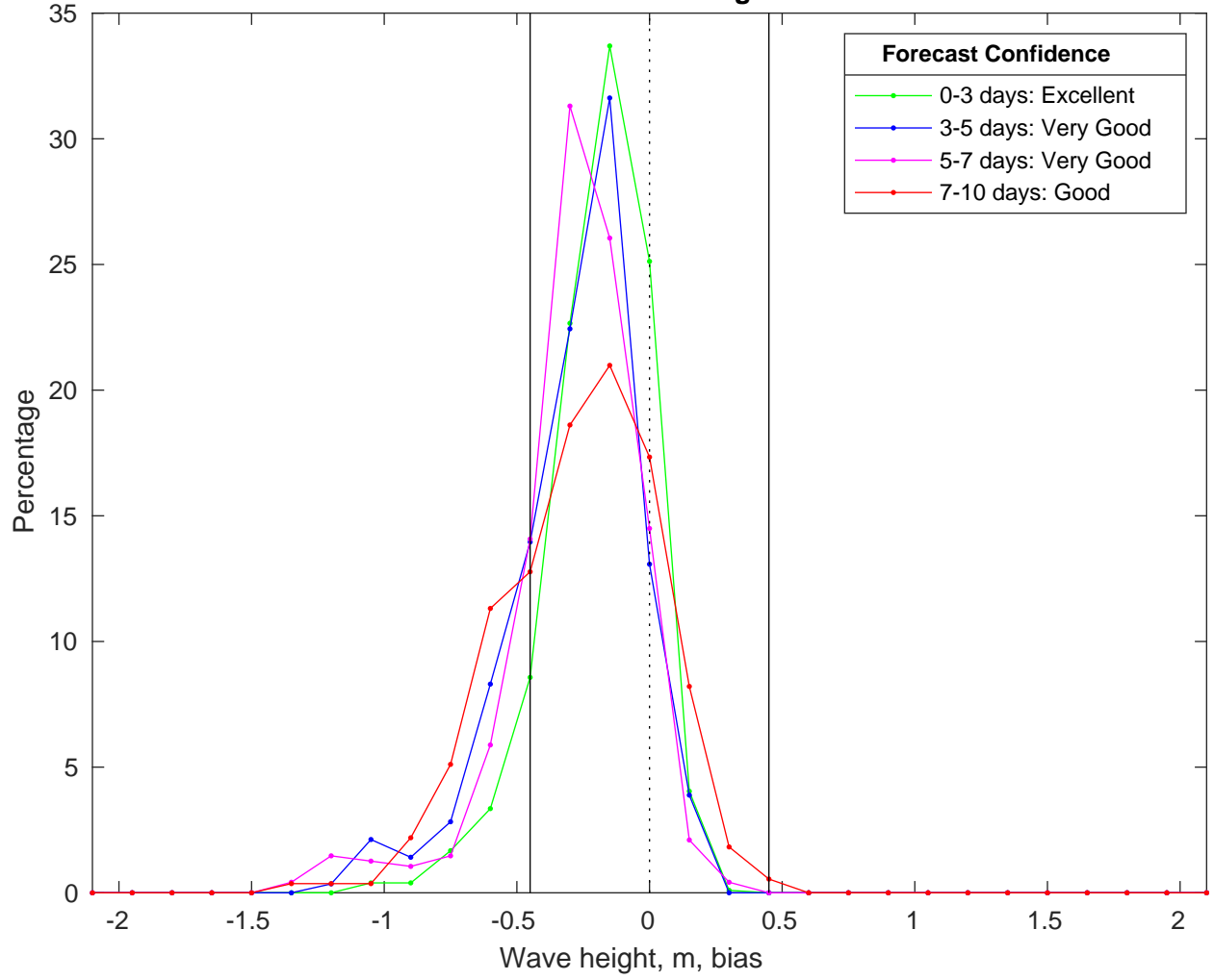
NDBC 52211 vs CMEMS Waves Bias Histogram: 08-Feb-2025
