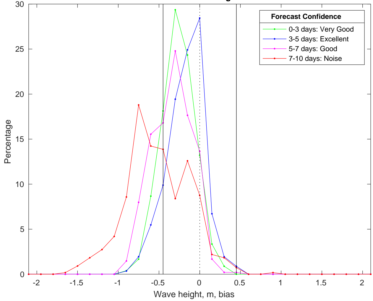
NDBC 52213 vs CMEMS Waves Bias Histogram: 08-Feb-2025
