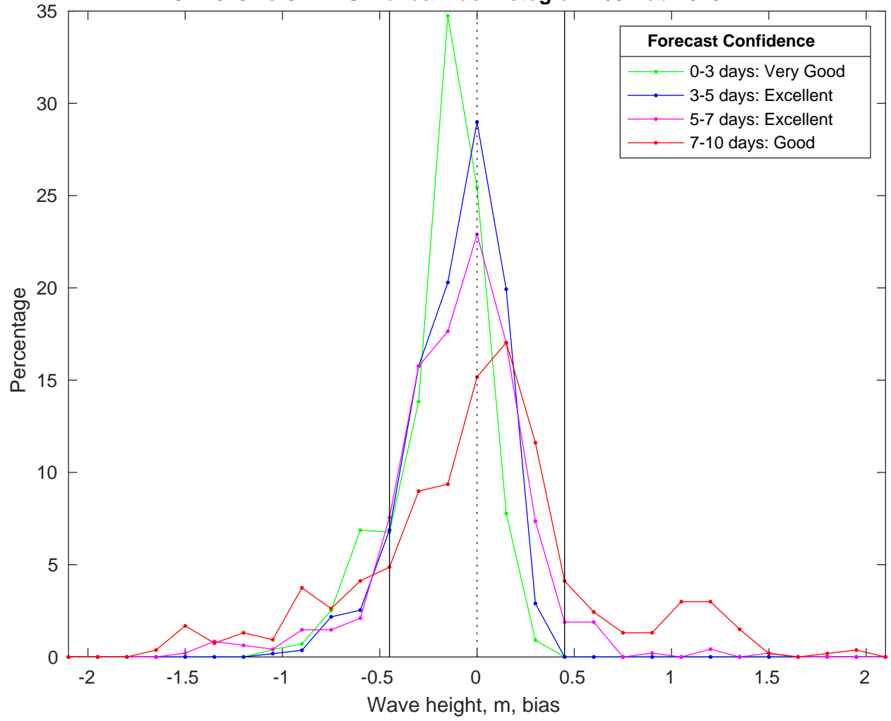
NDBC 42019 vs CMEMS Waves Bias Histogram: 09-Feb-2025
