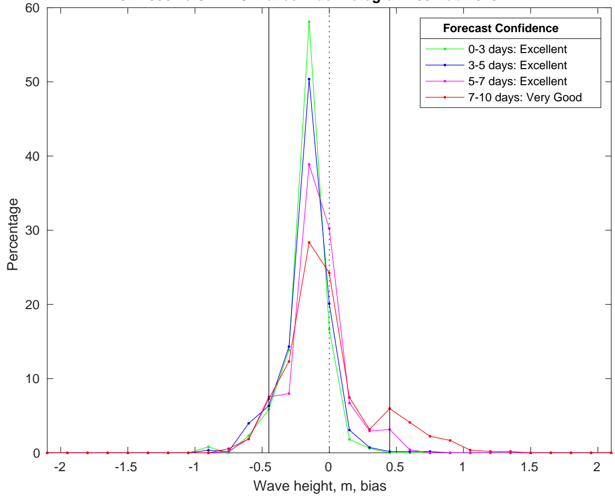
NDBC 42036 vs CMEMS Waves Bias Histogram: 09-Feb-2025
