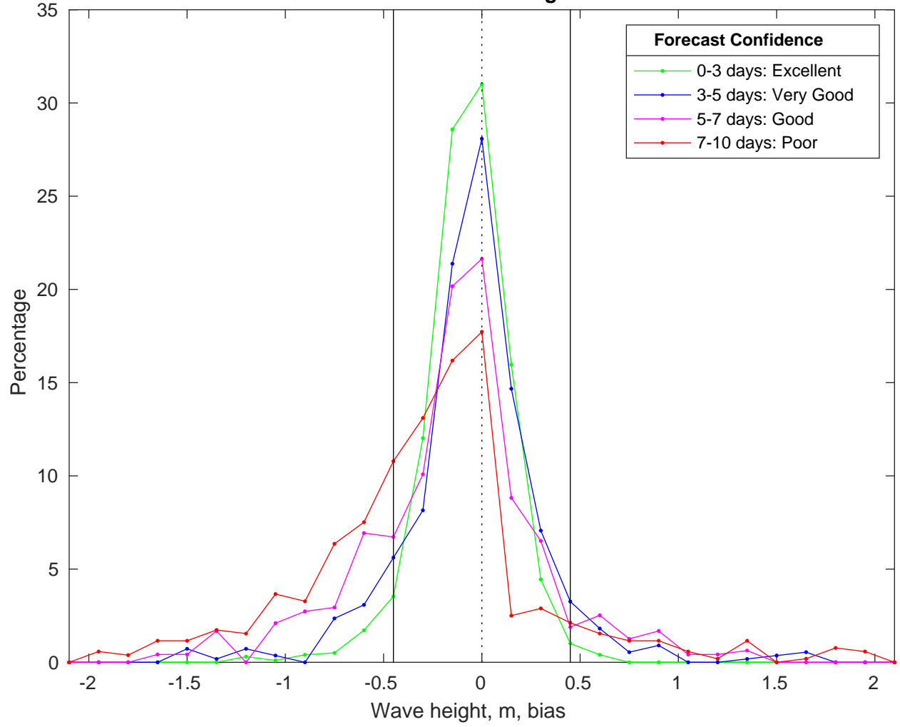
NDBC 46028 vs CMEMS Waves Bias Histogram: 09-Feb-2025
