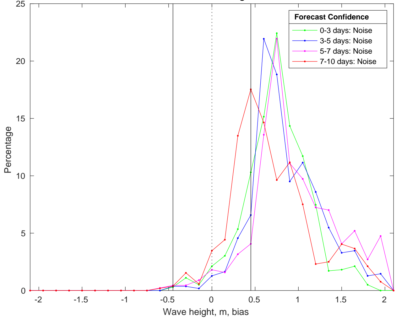
NDBC 46053 vs CMEMS Waves Bias Histogram: 09-Feb-2025
