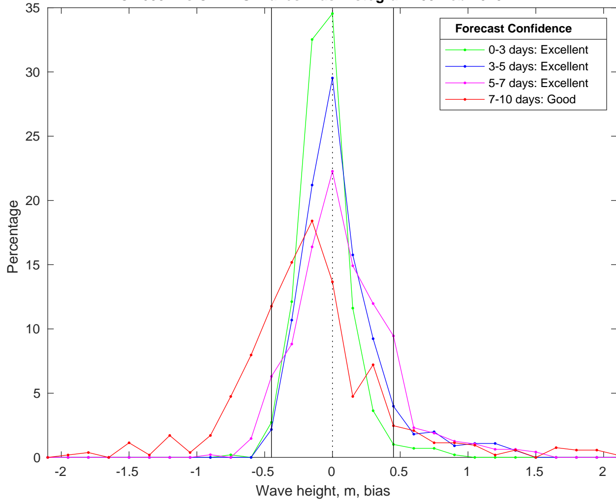
NDBC 46054 vs CMEMS Waves Bias Histogram: 09-Feb-2025
