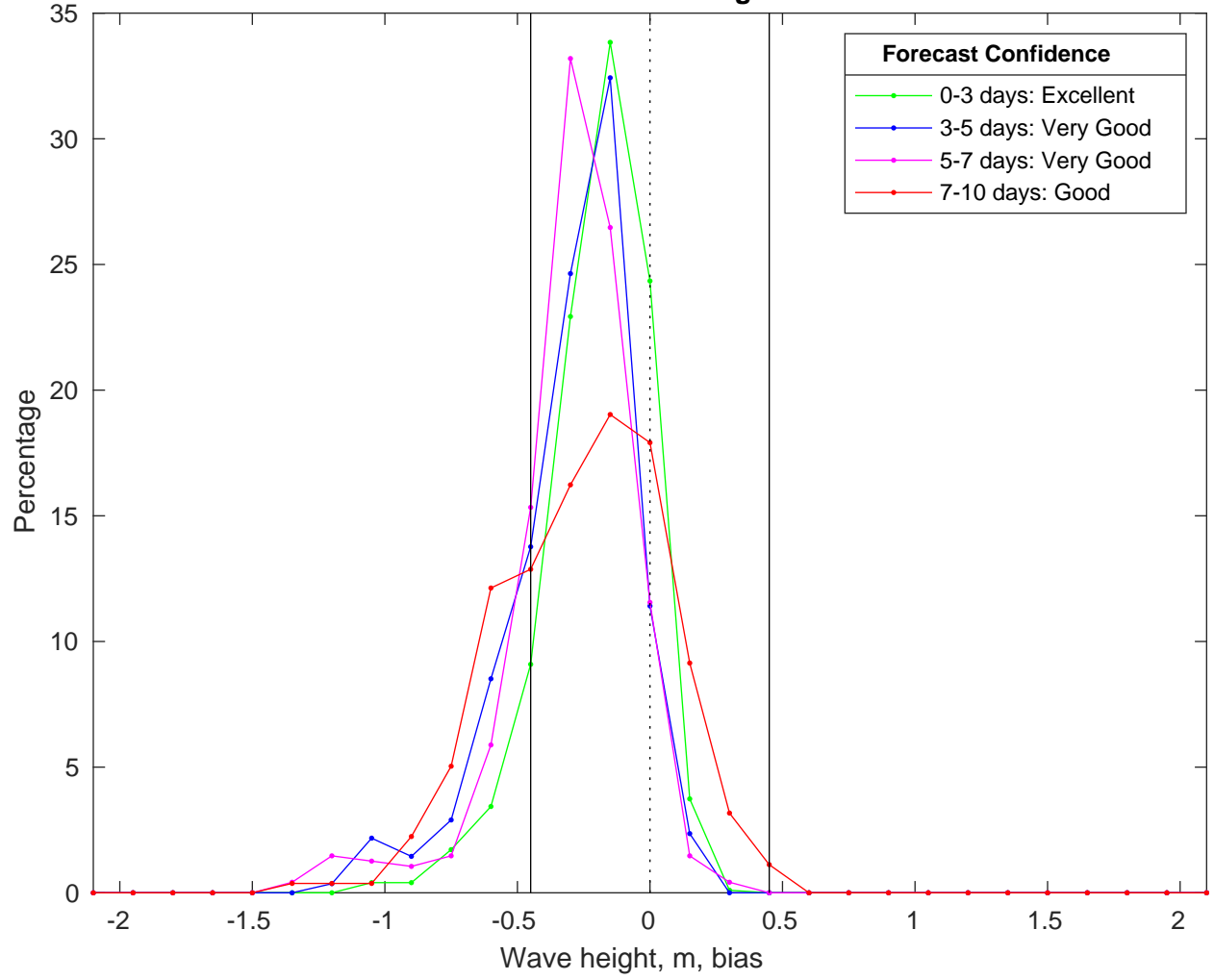
NDBC 52211 vs CMEMS Waves Bias Histogram: 09-Feb-2025
