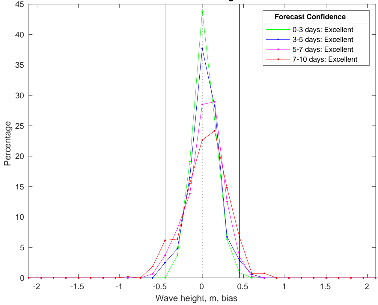
NDBC 41040 vs CMEMS Waves Bias Histogram: 11-Feb-2025
