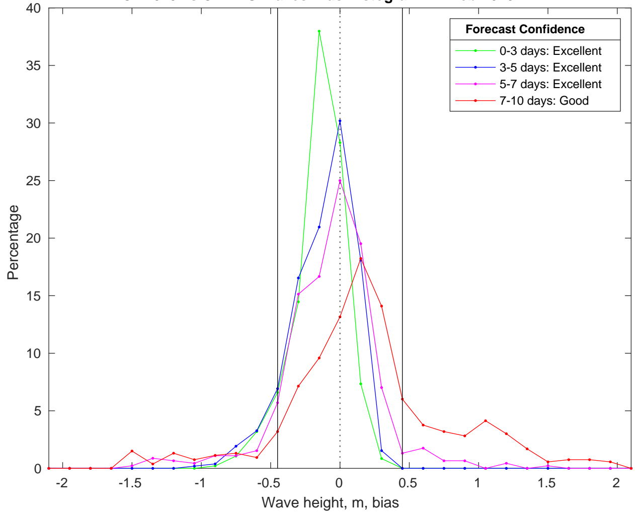
NDBC 42019 vs CMEMS Waves Bias Histogram: 11-Feb-2025
