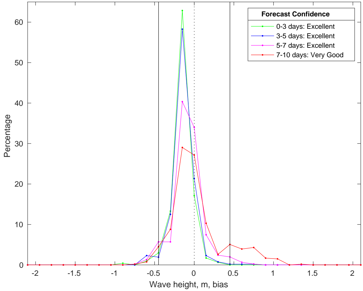
NDBC 42036 vs CMEMS Waves Bias Histogram: 11-Feb-2025
