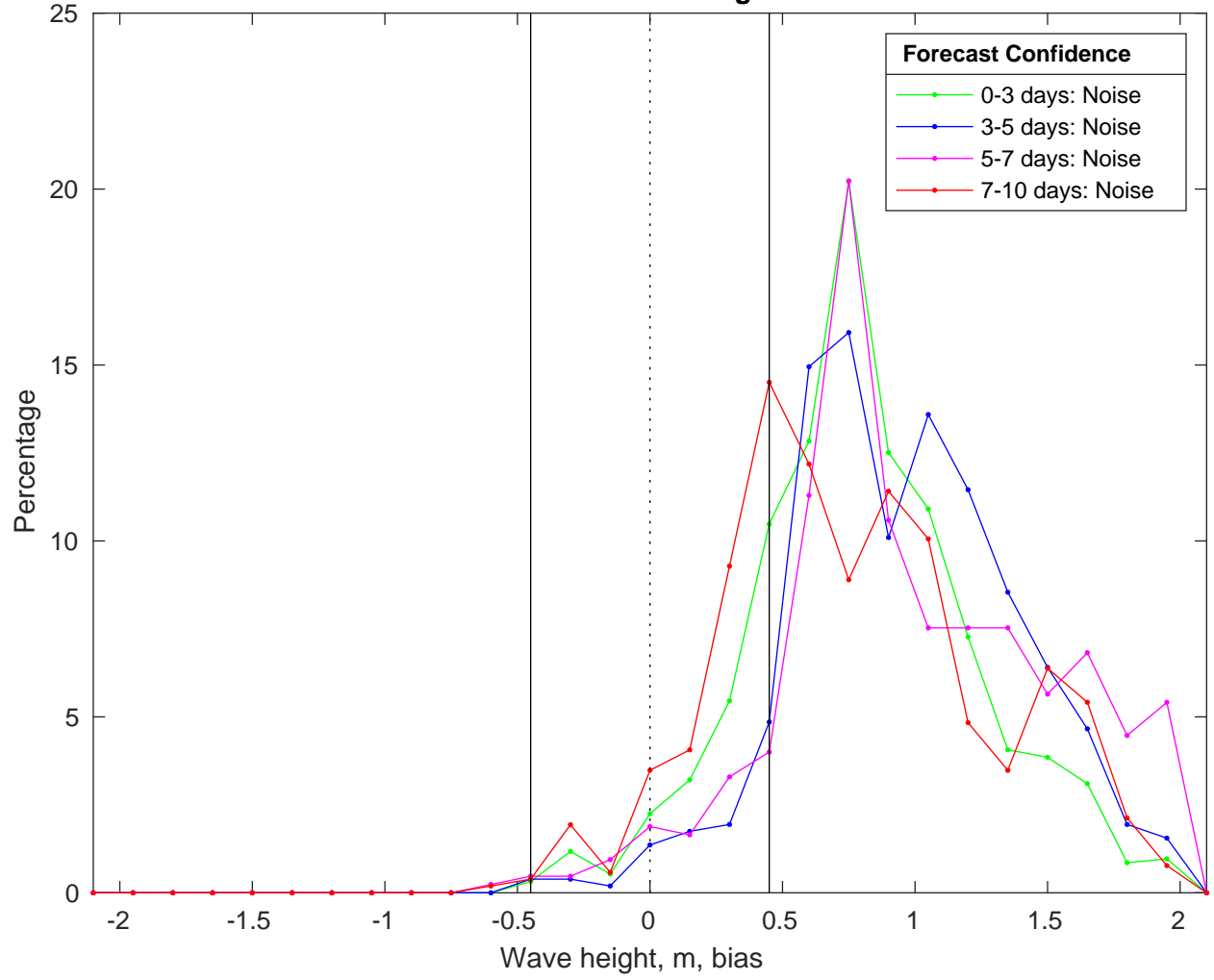
NDBC 46053 vs CMEMS Waves Bias Histogram: 11-Feb-2025
