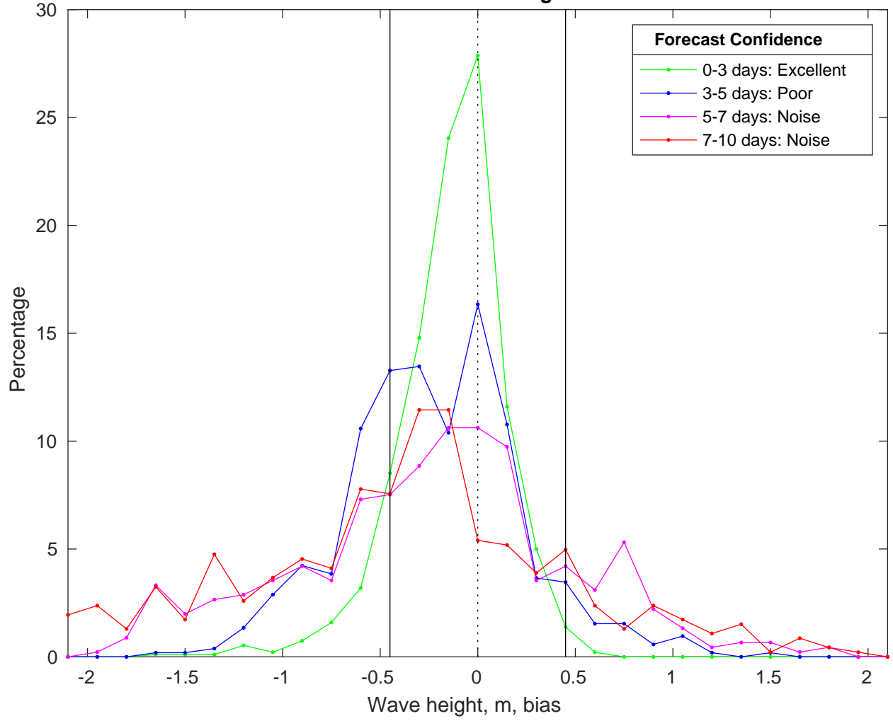
NDBC 46246 vs CMEMS Waves Bias Histogram: 11-Feb-2025
