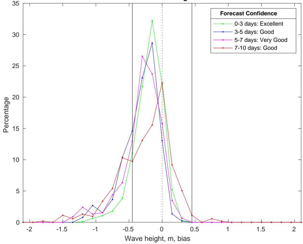
NDBC 52211 vs CMEMS Waves Bias Histogram: 11-Feb-2025
