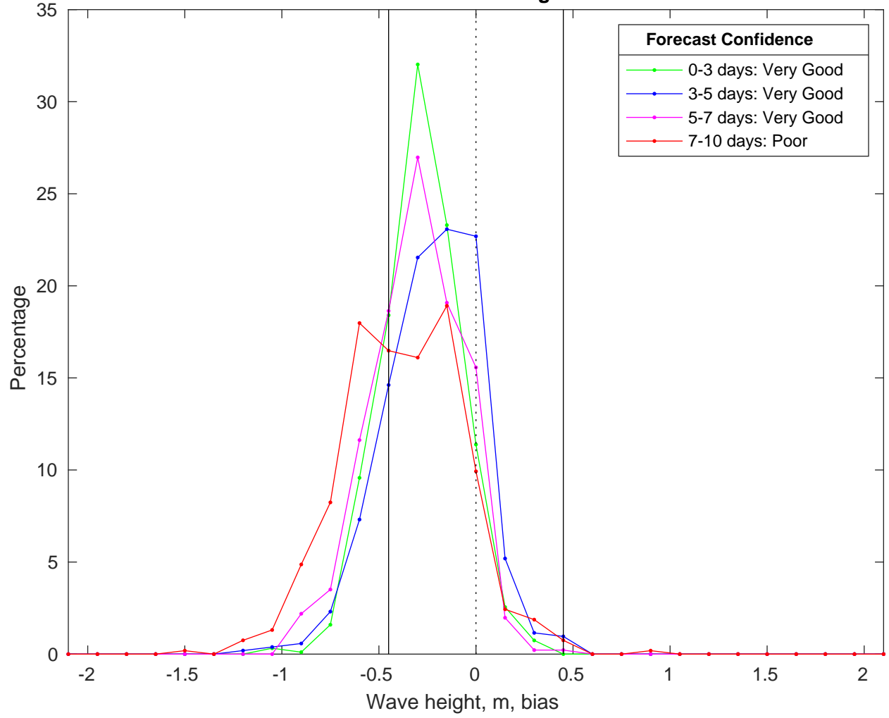
NDBC 52213 vs CMEMS Waves Bias Histogram: 11-Feb-2025
