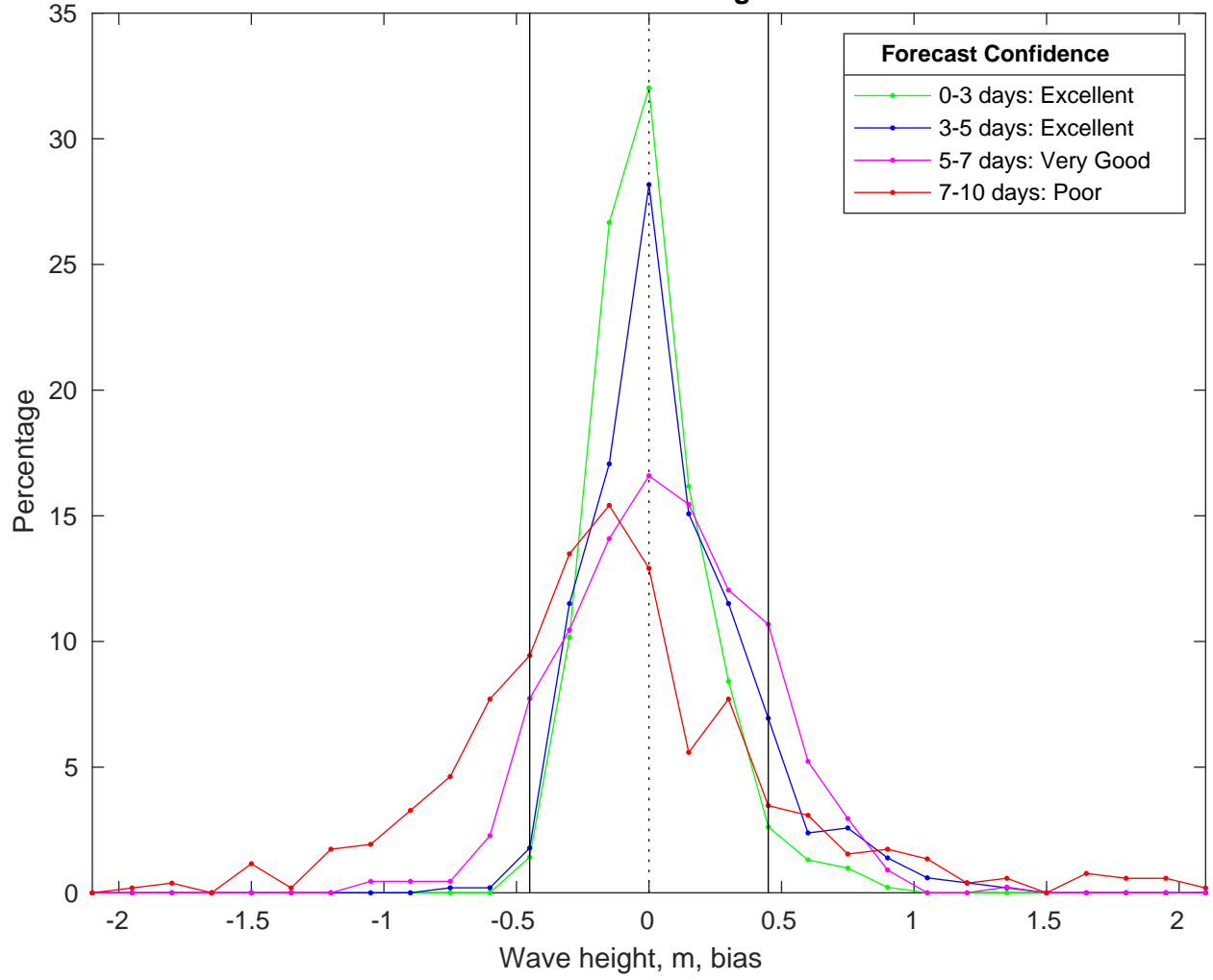
NDBC 46054 vs CMEMS Waves Bias Histogram: 12-Feb-2025
