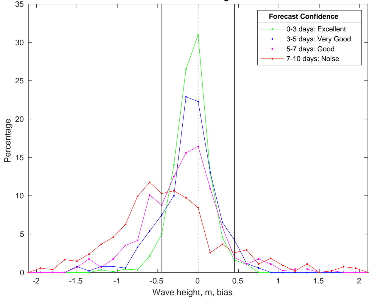
NDBC 46028 vs CMEMS Waves Bias Histogram: 13-Feb-2025
